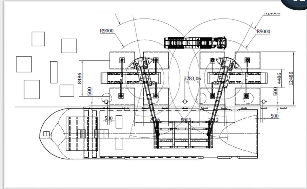
Simulación 2D – Izaje de Carga Sobredimensionada
